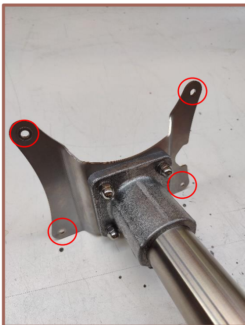
Instructie 2: Patroon van de montageplaat
